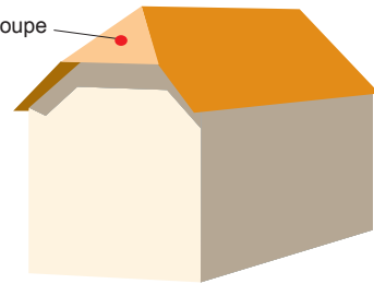
toit à longs pans brisés et croupe
