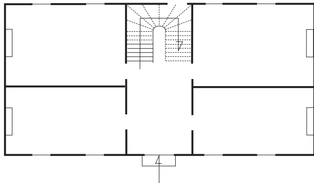
une variante : maison double en profondeur avec couloir
